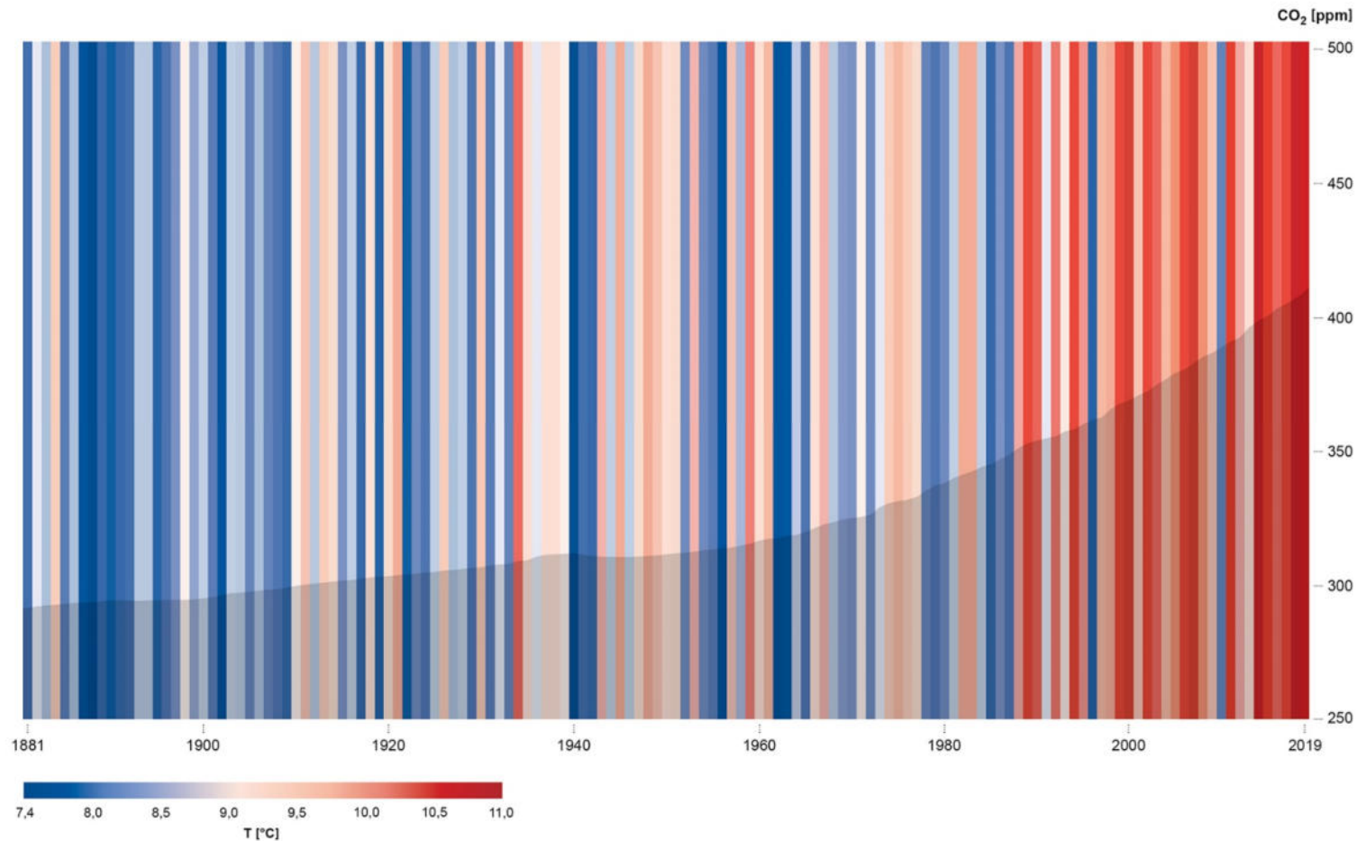
Warming Stripes NRW – Barcode des Klimawandels
