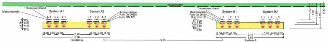
Prinzipische der Lage der Leerrohre/Erdkabel nach Abschluss der Baumaßnahme (Detaildarstellung 1:75; Amprion GmbH, 7/2011)
